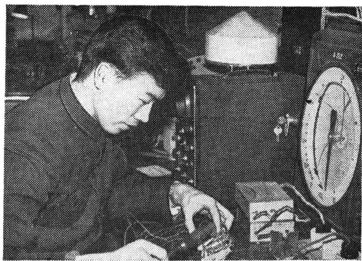
Студент 643-й группы Бянь Нан-хуа под руководством доцента А. А. Сивкова успешно разрабатывает тему своего дипломного проекта «Малогабаритный оптико-акустический газоанализатор». Наш фотокорреспондент Зинаида Степанова запечатлела китайского студента за работой.
