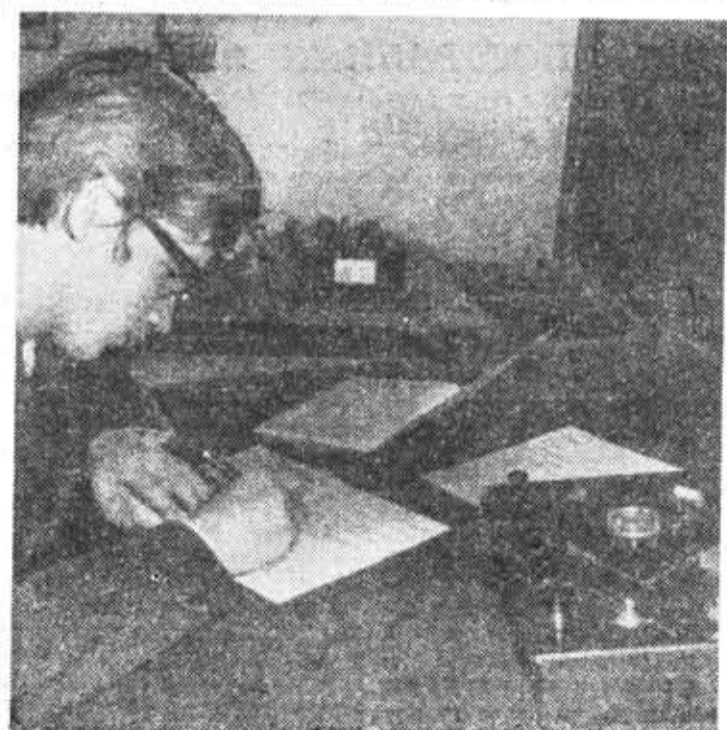
Николай Полевой, студент второго курса, измеряет емкость конденсаторов при помощи баллистического гальванометра. Фото З. САНИНОЙ
