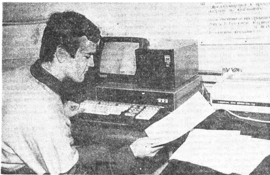
Студент 541-й группы Михаил Чернышев выполняет на кафедре спектральных и оптико-физических приборов учебно-исследовательскую работу «Исследования плазмы методом резонансных флуоресценций». Фото Э. Степановой
