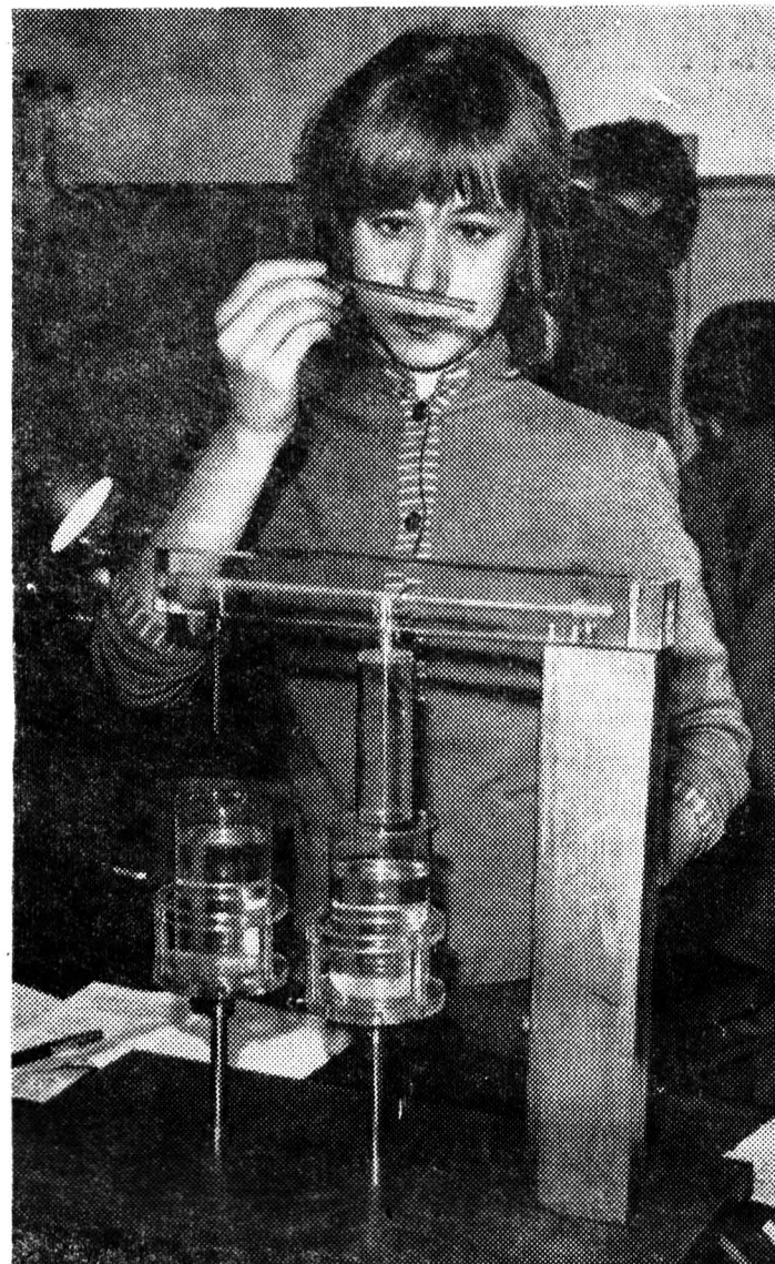
Лабораторные занятия на кафедре физики. Студентка 200-й группы Наташа Захарова определяет коэффициент поверхностного натяжения жидкости. Задание, знакомое еще по школьным урокам, но выполнять его в институте несравненно сложнее.
