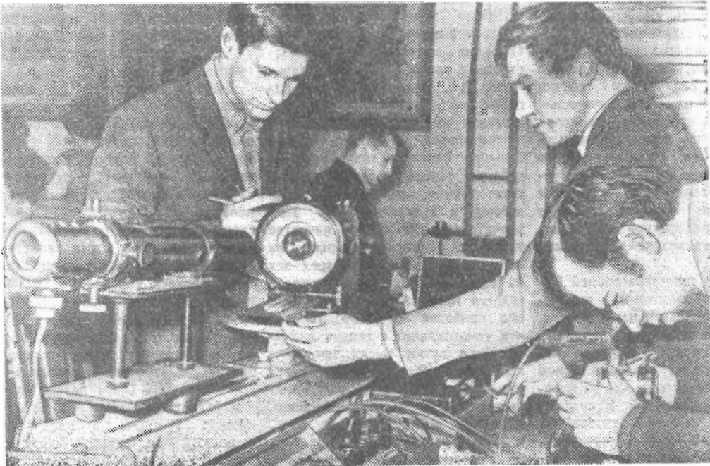
Лабораторная работа по курсу «Оптические измерения». Студенты 436-й группы Геннадий Капустин, Юрий Куржой и Юрий Федоров измеряют радиусы кривизны линз методом Гюйона.
