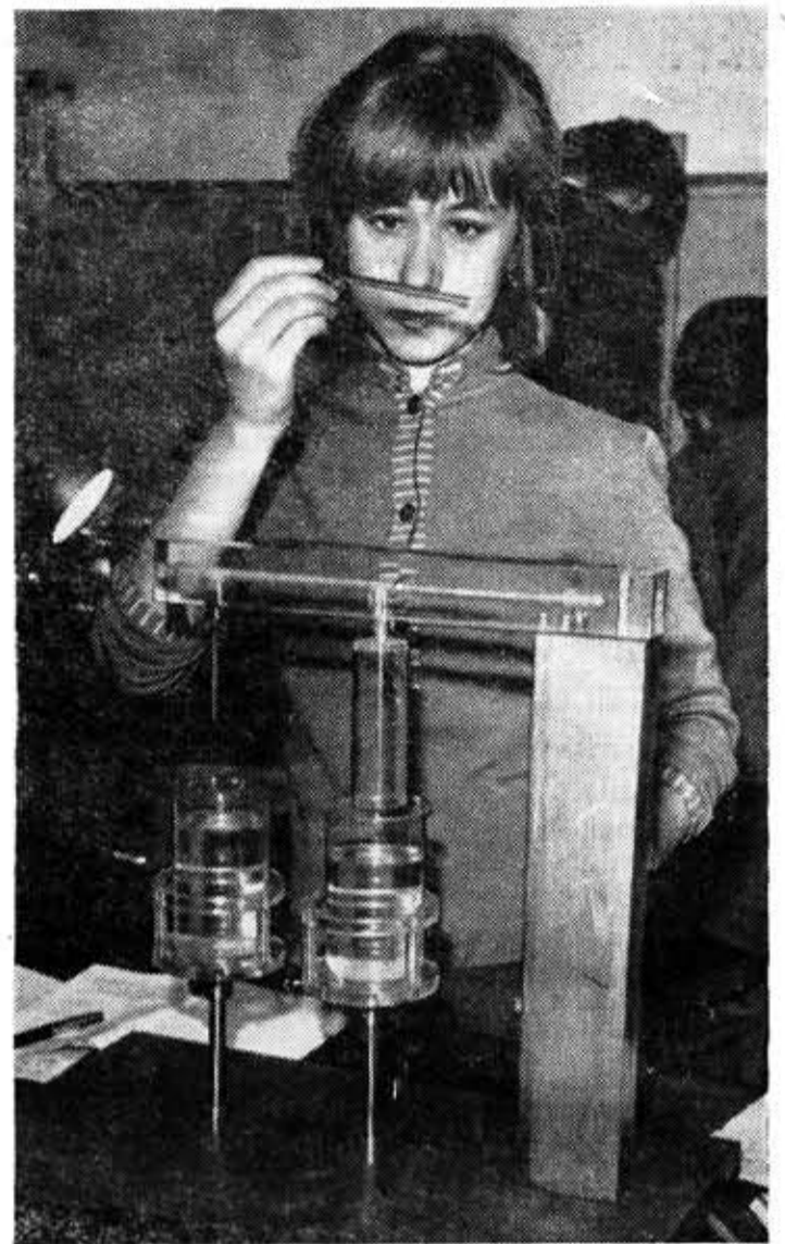
Лабораторные занятия на кафедре физики. Студентка 200-й группы Наташа Захарова определяет коэффициент поверхностного натяжения жидкости. Задание, знакомое еще по школьным урокам, но выполнять его в институте несравненно сложнее.
